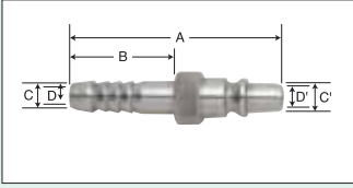
エアジョイントプラグ No.35P
