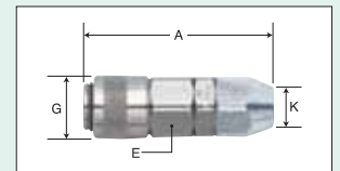
ミニエアジョイントソケット No.2SN
