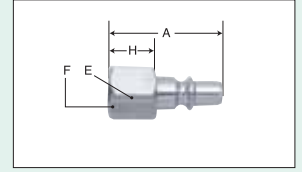
内ネジプラグ No.32P
