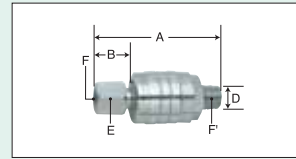
エアジョイントセット No.34
