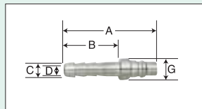
ミニエアジョイントプラグ No.2PH
