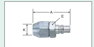
ミニエアジョイントプラグ No.2PN
