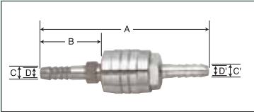
エアジョイントセット No.26
