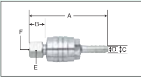
エアジョイントセット No.32
