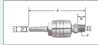
エアジョイントセット No.28
