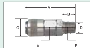
ミニエアジョイントソケット No.2SM
