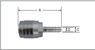
エアジョイントソケット No.26S
