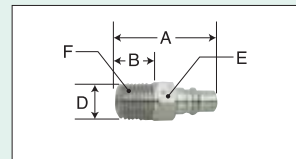
ミニエアジョイントプラグ No.2PM
