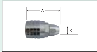
エアジョイントソケット No.35S
