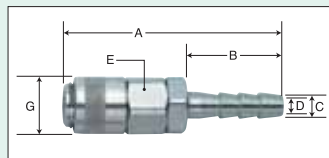
ミニエアジョイントソケット No.2SH
