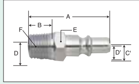
エアジョイントプラグ No.28P
