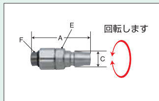
エアースタースターガン用プラグ
