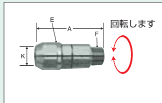
ウレタンホース専用金具 サイズR1/4
