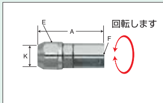
ウレタンホース専用金具 サイズRC1/4
