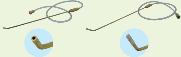
D-5用 オプションノズル D-5 別作ALノズル ●全長(mm)：350 ●質量(g)：224
