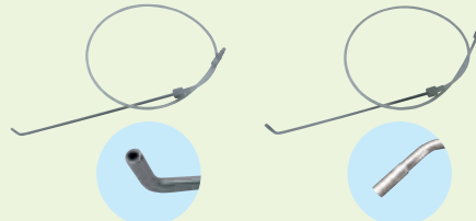
D-7用 オプションノズル D-7 別作APLノズル ●全長(mm)：340 ●質量(g)：146
